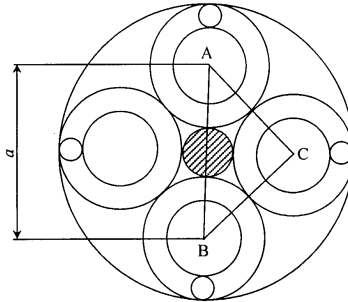
Рис. 3.2. Диаметр элементарной группы кабеля
