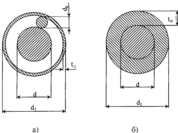
Рис. 3.1 Диаметр изолированной жилы
