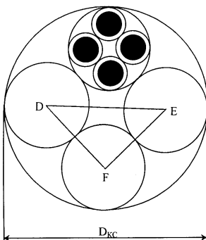
Рис. 3.3. Диаметр кабельного сердечника 4x4
