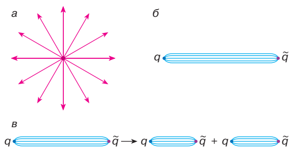
Рис. 2. Схема силовых линий электрического поля в электростатике (а) и глюонного поля между кварком и антикварком (б), а также схема разрыва жгута при его большом растяжении (в)
