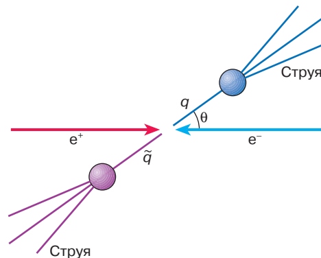
Рис. 4. Схема рождения двух кварковых струй в реакции e^+ + e^- \rightarrow \gamma_{\text{вирт}} \rightarrow q + \bar{q} .
